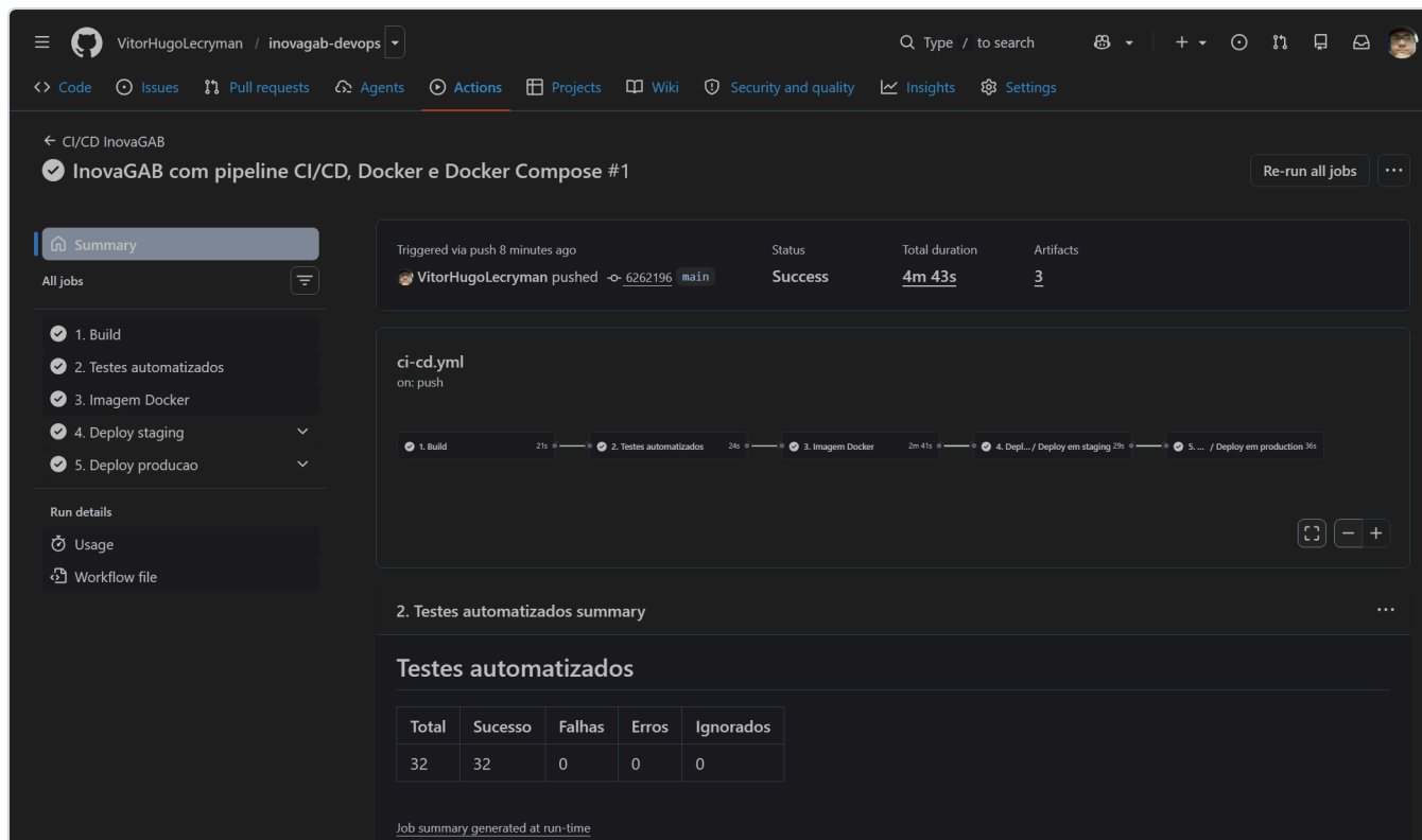
Figura 3 — Testes automatizados executados no pipeline.
