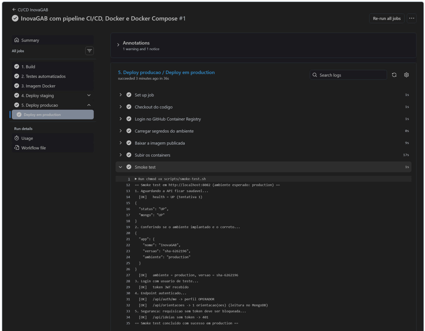
Figura 6 — Deploy em produção: ambiente: production e smoke test aprovado.
